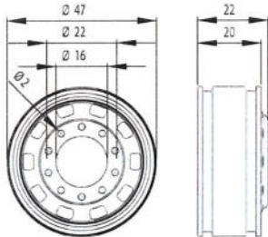
01 Felge schmal Aluminium 2 11000048
